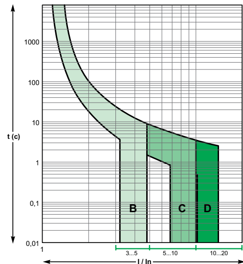
Криві відключення
