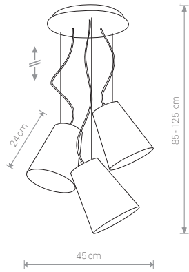
RETTO A abazur, stal lakierowana / shade, painted steel / абажур, лакированная сталь 5197 3×E27, max 60W
