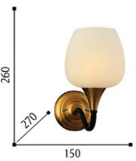
4590-11 ↑ 150 ↑ 260 ↑ 270 ↓ E14 220V 1 x 40W IP20 metal, glass
