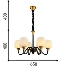
4590-46 Ø 650 ↑ 800 ↓ E14 220V 6 x 40W IP20 metal, glass
